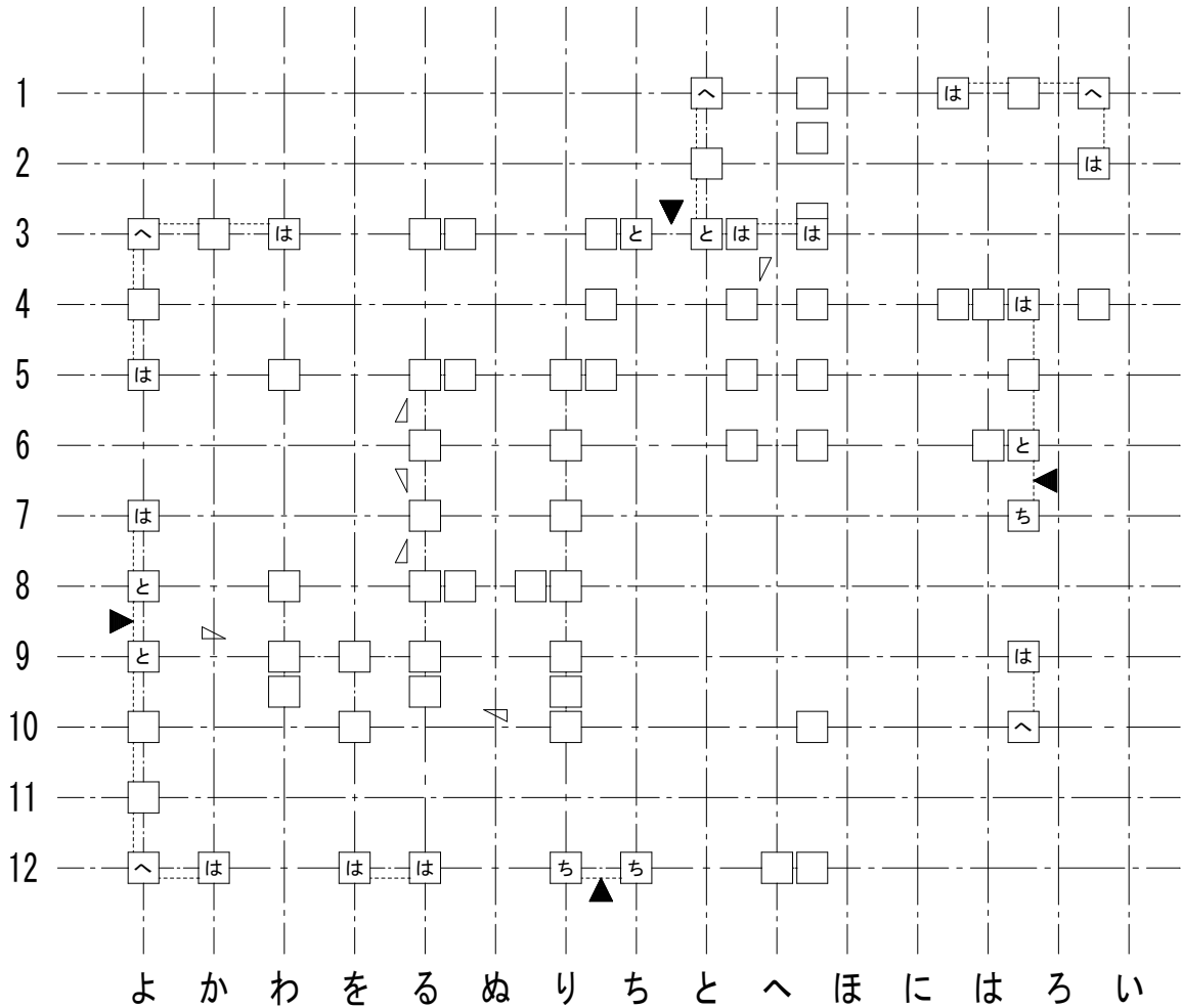
1 階柱壁伏図
